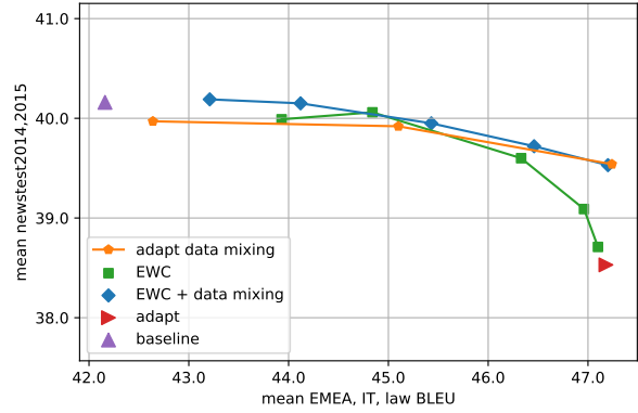
(b) EN→FR
